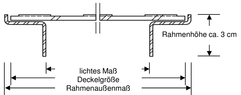
Systemschnitt
